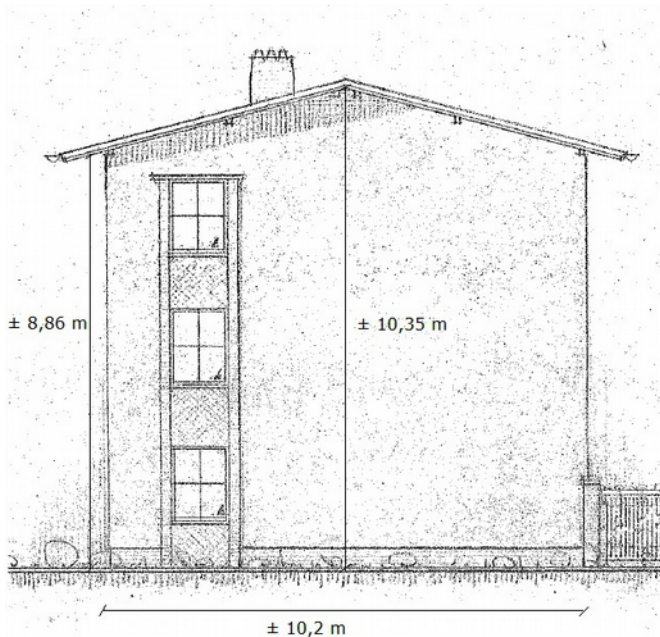
Afmetingen renovatiegevel Snipstraat, Pluivierstraat, Kokmeeuwstraat en Roerdompstraat
